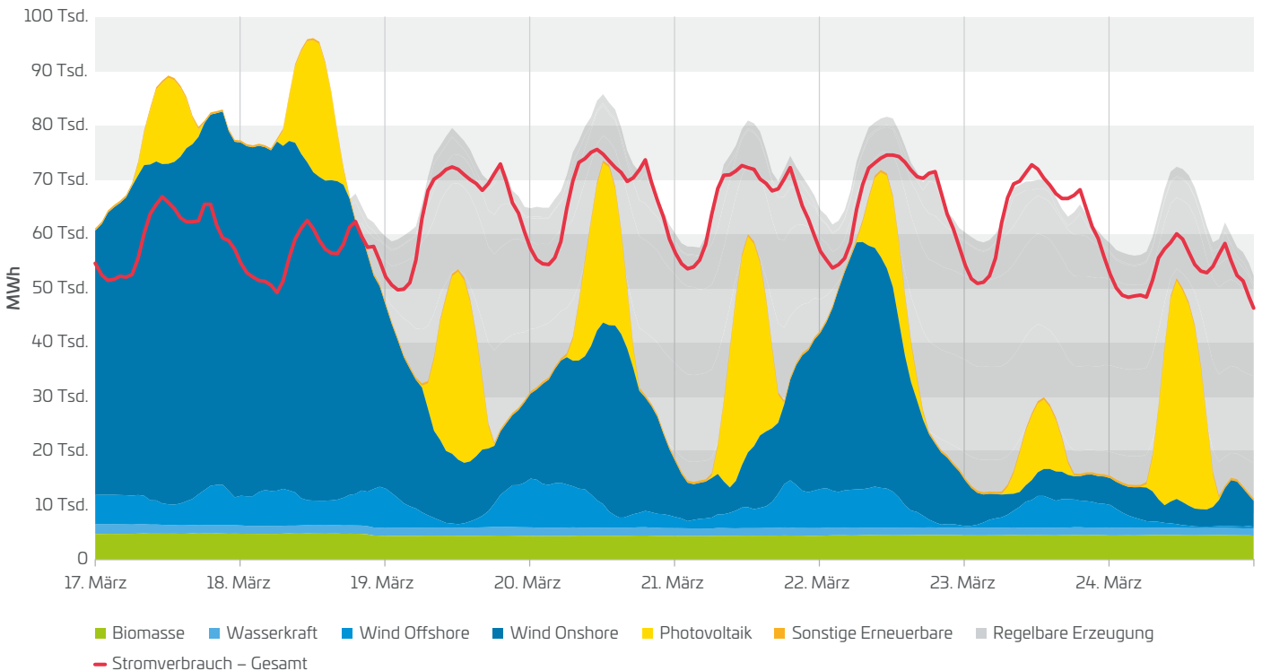
Abb. 2 Residuallast bei 65 % EE (Ziel 2030): Das Maximum ist fast gleich hoch wie heute, aber nur noch an 6.500 Jahresstunden wird konventionelle Erzeugung benötigt (Quelle: SMARD Strommarktdaten der Bundesnetzagentur, Skalierung der fluktuierenden Energien: Flexperten)
