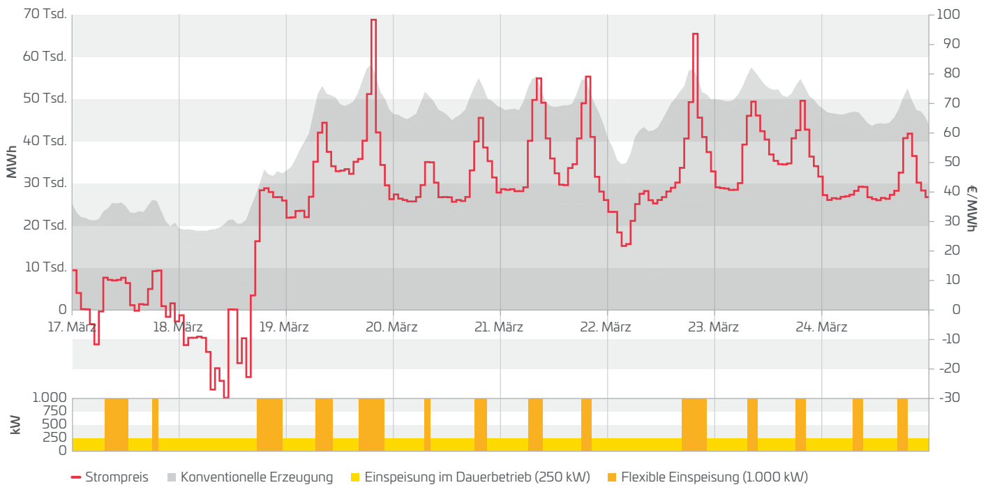
Abb. 3 | Marktintegration durch Direktvermarktung: Residuallast, Spotmarktpreise der EPEX-Auktion und typische BHKW-Einspeisung bisher – und in Zukunft in Zusammenarbeit mit dem Direktvermarkter (Quelle: SMARD Strommarktdaten der Bundesnetzagentur; Beispielfahrplan: Flexperlen)
